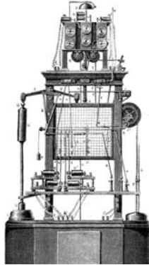
Meteorológiai adatokat rögzítő készülék (1873)
