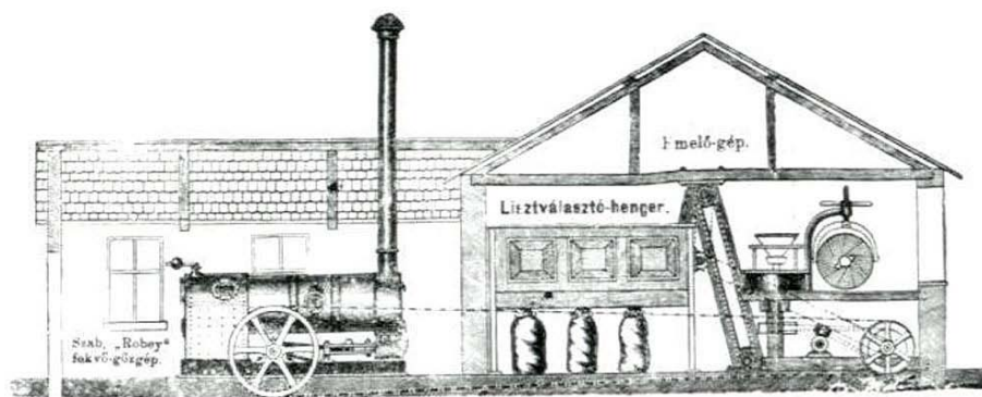
Kisebb gőzmalom rajza (mozgatható gőzgéppel) 1884-ből
