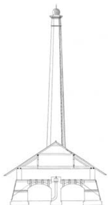
Az eredeti körkemence metszete
