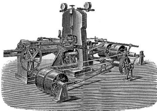
Donga- és fenékkilésző gép az 1880-as években
