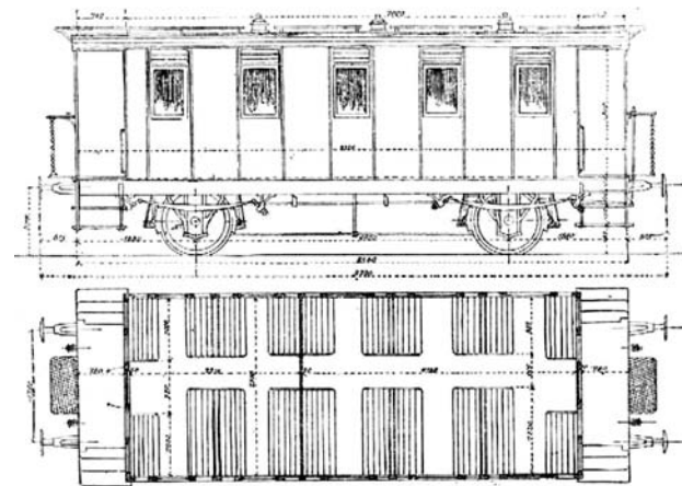
A Déli Vasút két (az egyik I. és II. osztályú, a másik III. osztályú) személyszállító vagonja 1896-ban és az ülések elrendezése
