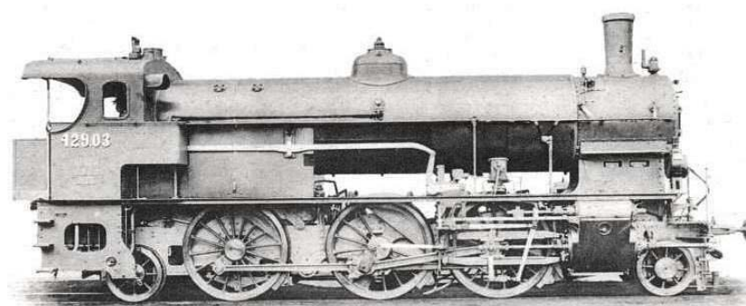
A Déli Vasút 429. sor. Prairie-jellegű 2 hengerű mozdonya. Építette a Magyar Királyi Államvasutak Gépgyára Budapesten 1911/12. Prairie Type der Personenzuglokomotive der Süd-Bahn. Serie 429. Gebaut von der Maschinenfabrik der königl. Ungarischen Staatsbahnen zu Budapest 1911/12.
