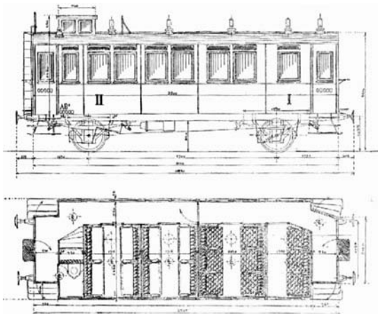
A Déli Vasút két (az egyik I. és II. osztályú, a másik III. osztályú) személyszállító vagonja 1896-ban és az ülések elrendezése
