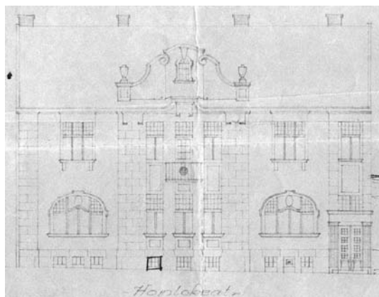
A homlokzat terve
